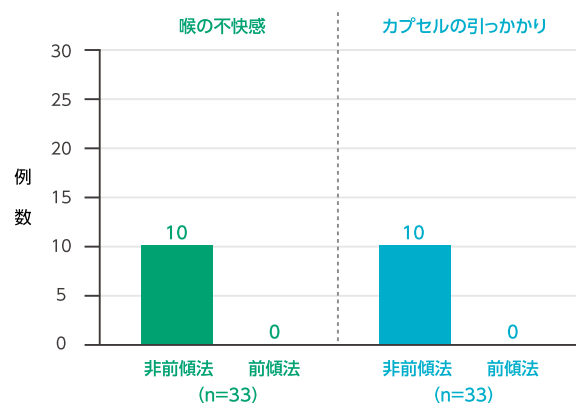
b. 前傾法によるカプセル嚥下時の変化
